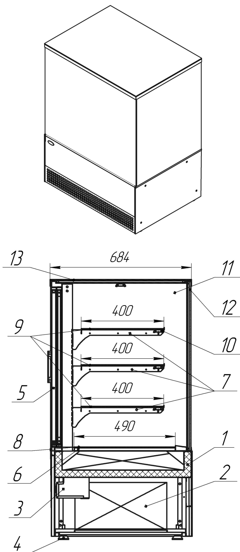
Схема сборки SIGMA CUBE – IN (695)
